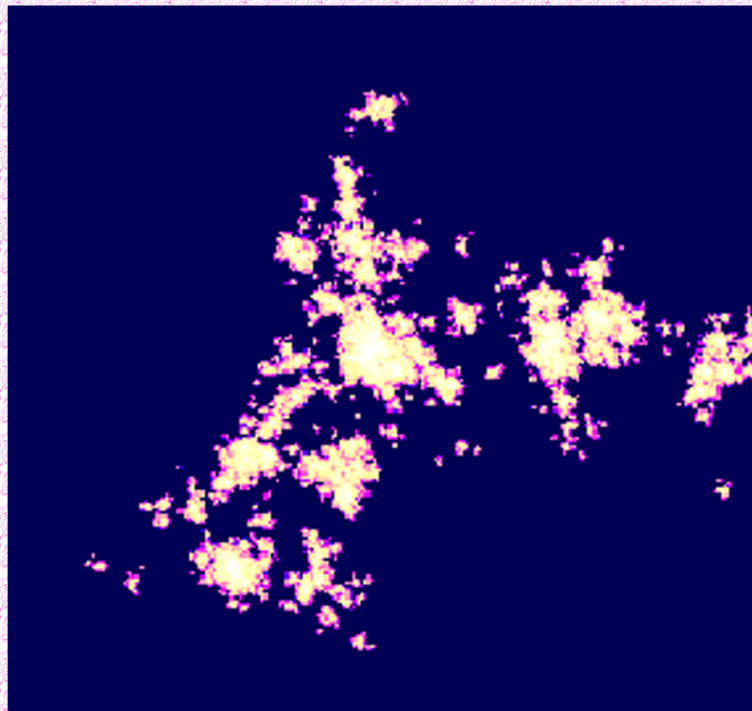
Pfenniger & Combes 1994
