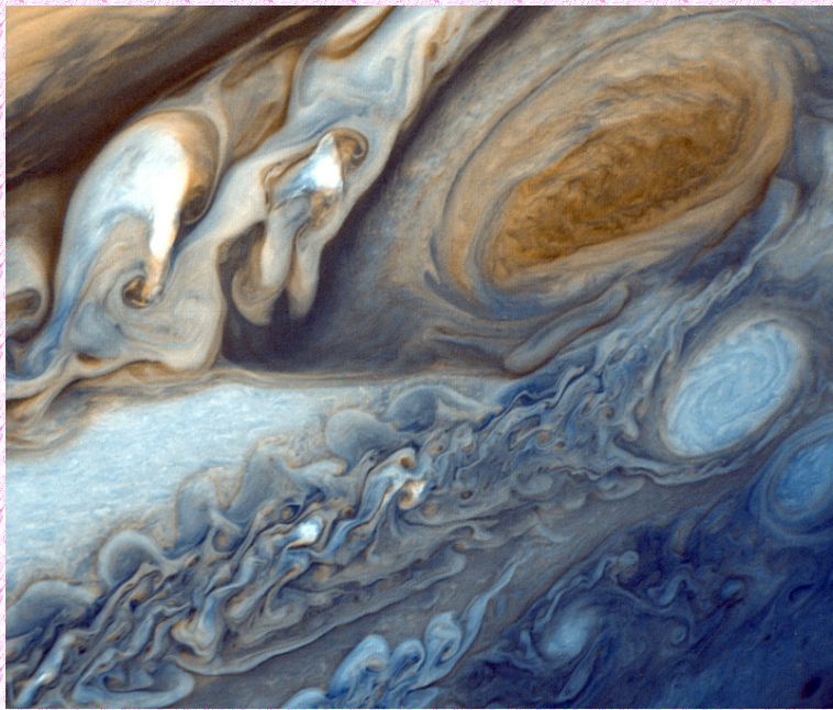
JPL-NASA Voyager 1
