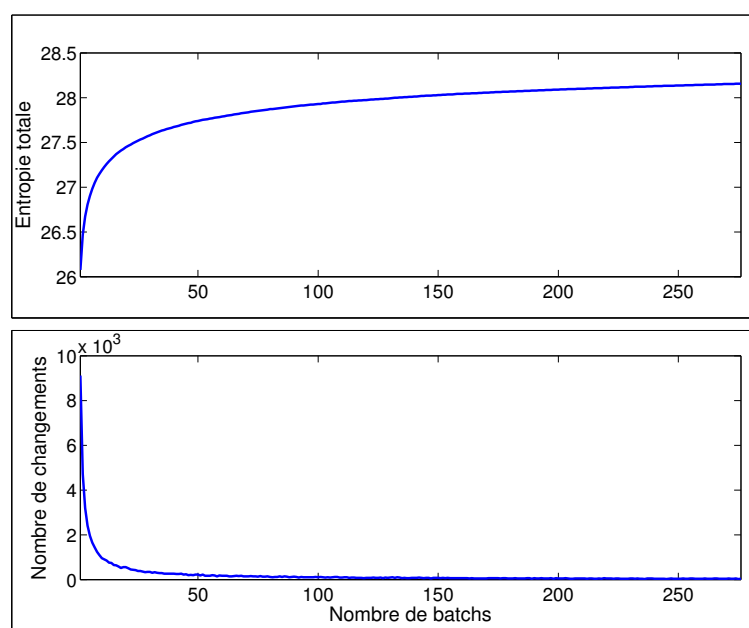
FIGURE 6.3 – De haut en bas : (A) évolution de l’entropie de la base échantillonnée en fonction du nombre de batches de 100.000 échantillons pris en compte ; (B) Nombre de profils différents dans la nouvelle base échantillonnée après chaque batch.
