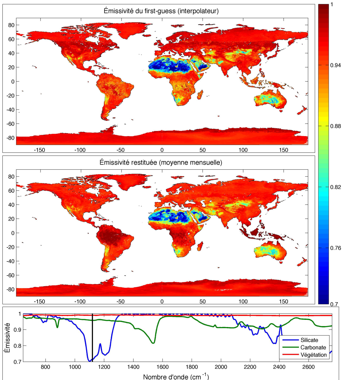
FIGURE 3.4 – Émissivité moyenne en janvier à 1120\text{ cm}^{-1} , la première ébauche interpolée à partir des émissivités de MODIS est en haut, les émissivités restituées sont au centre. Les trois spectres du bas représentent des spectres d'émissivité correspondant à des sols arides (silicates en bleu et carbonates en vert) et à un sol végétalisé (en rouge).
